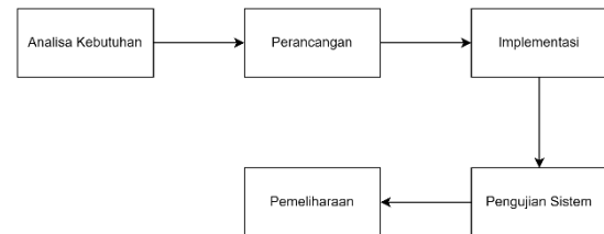
Gambar 2. Tahapan Penelitian
