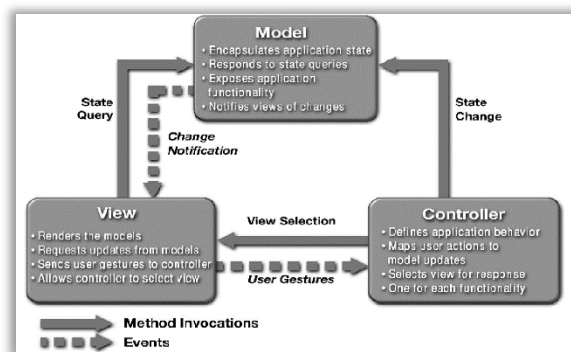
Gambar 5 Arsitektur MVC
