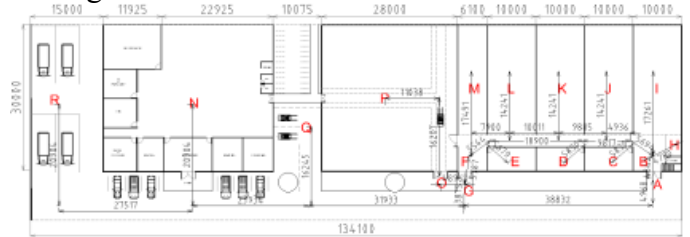
Gambar 8. Jarak Perpindahan Antar Ruang Layout Usulan Gudang PT. MKM
